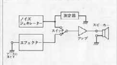
図2 ノイズレベルの測定法(聴感比較法)
