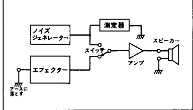
図2 ノイズレベルの測定法(聴感比較法)
