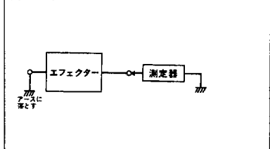
図2 ノイズレベルの測定法(聴感比較法)
