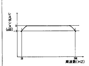
図3 周波数特性
